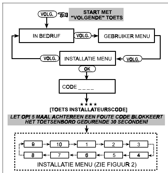
Figuur 1. In het installateursmenu komen
