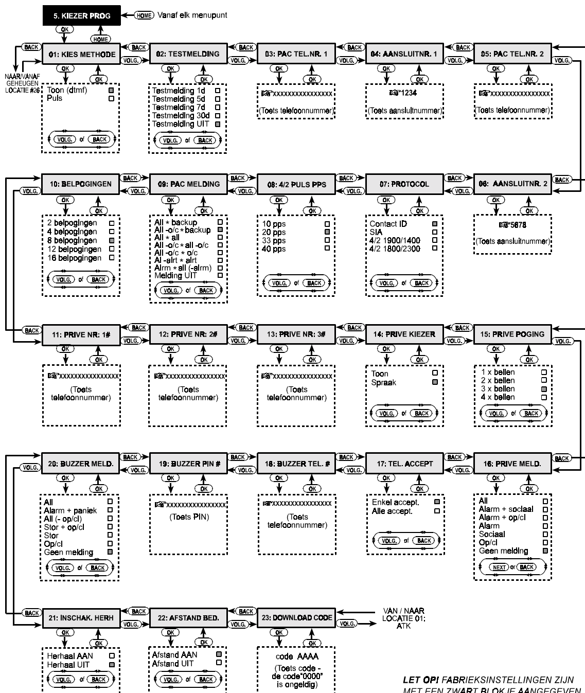
Figuur 5. KIEZERPROGRAMMERING flow diagram
