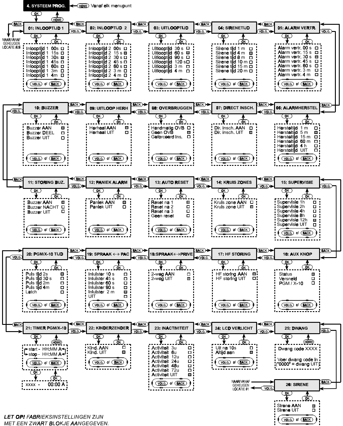
Figuur 4. SYSTEEM PROGRAMMERING flow diagram
