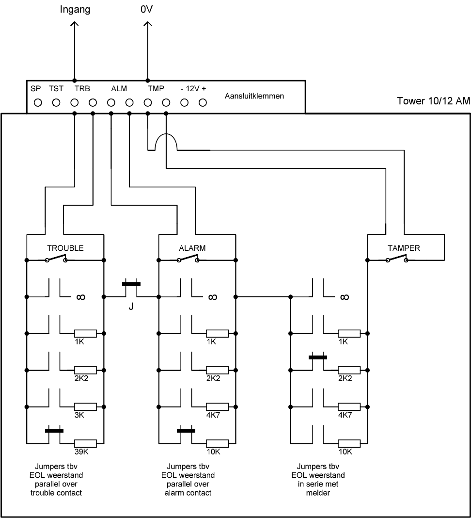
Tower 10 AM & Tower 12 AM aansluitschema (met EOL weerstanden)
