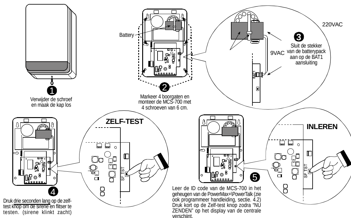
Figuur 3 – Installatie, testen en inleren
