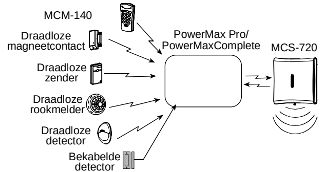
Figuur 2 - Integratie met een Alarmsysteem.
