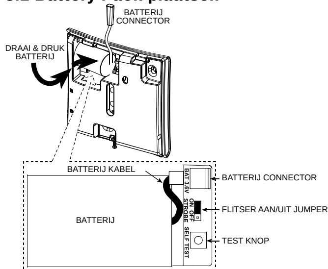
Figuur 4 - Battery Pack plaatsen
