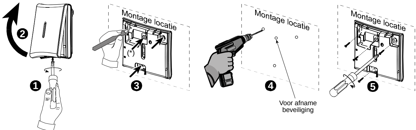
Figuur 3 - Installatie
