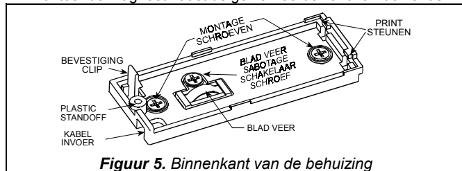
Figuur 5. Binnenkant van de behuizing
