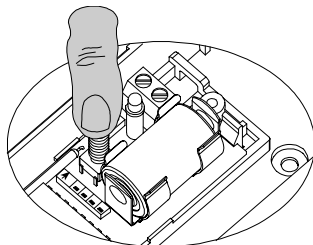
Figuur 8. De batterij op zijn plaats
