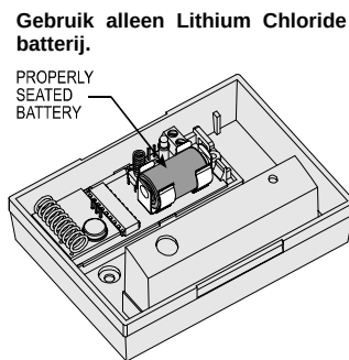
Figuur 8. De batterij op zijn plaats
