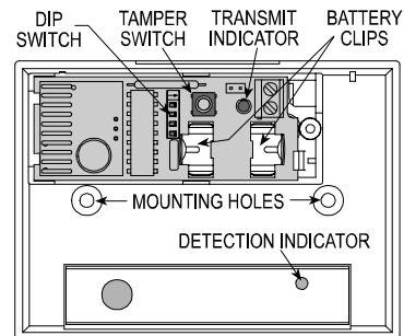
Figuur 5. Binnenkant van de MCT-501
