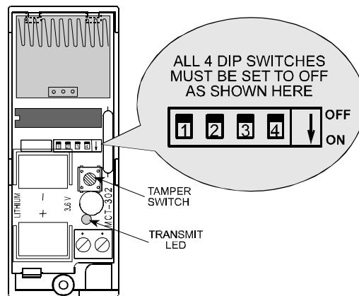
Figuur 6. DIP schakelaars – juiste positie
