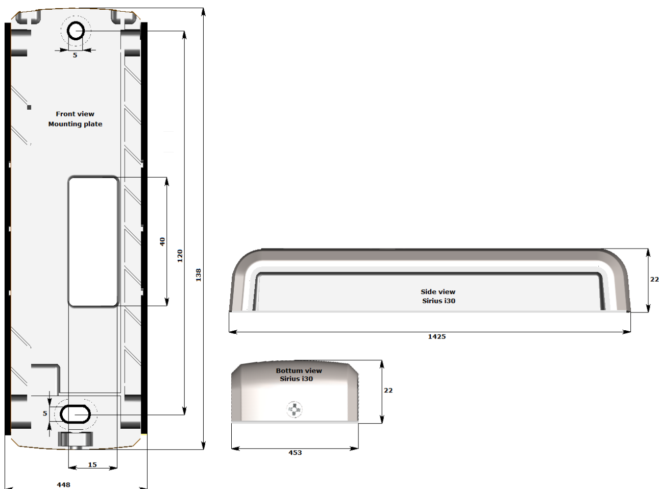
Afbeelding 1: Sirius i30 afmetingen
