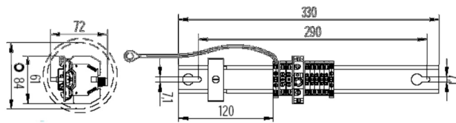
Aansluitblok
